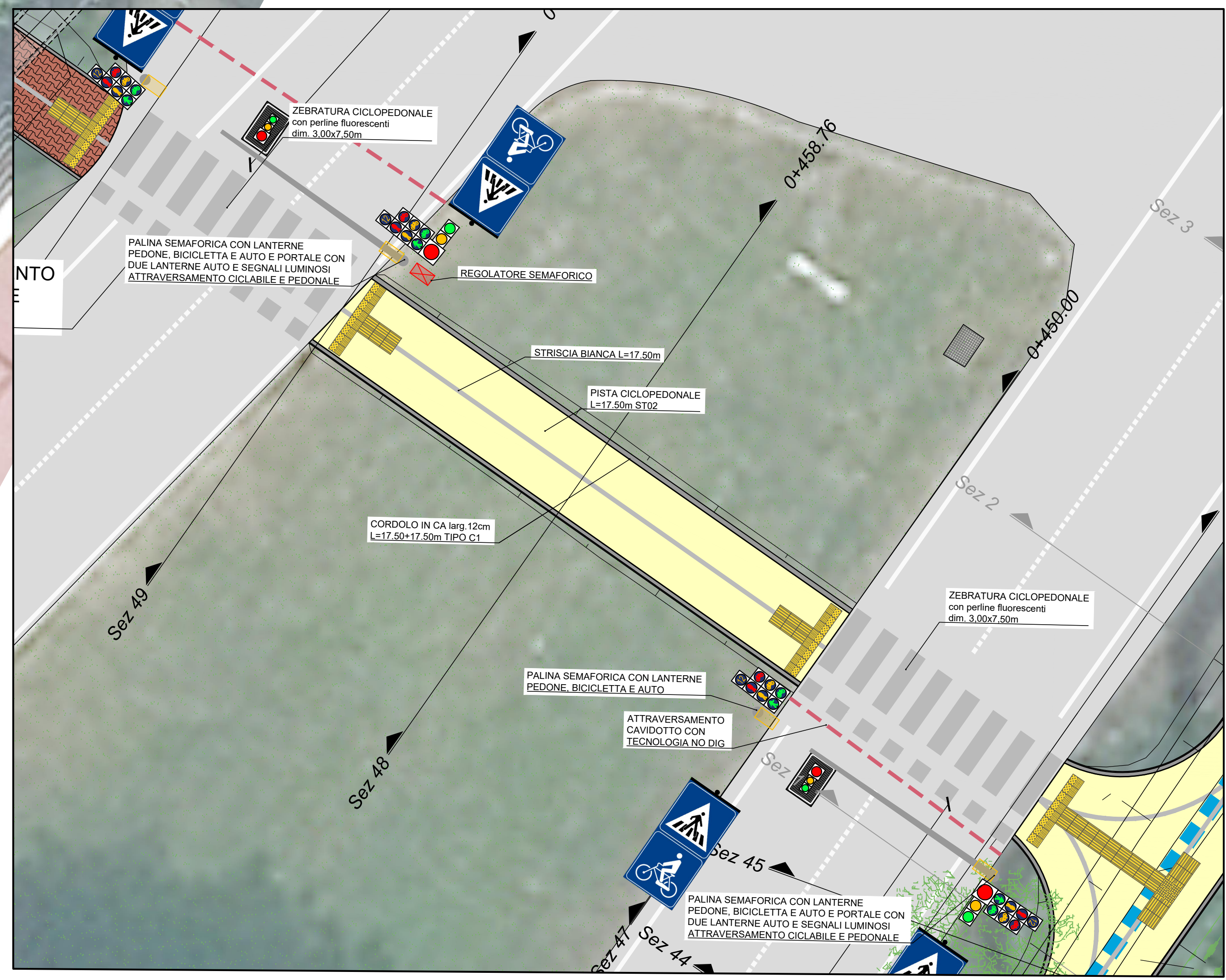
INGRANDIMENTO 1 scala 1:100
