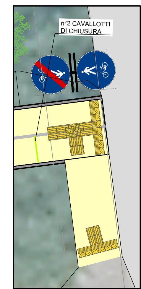
INGRANDIMENTO 2 scala 1:100
