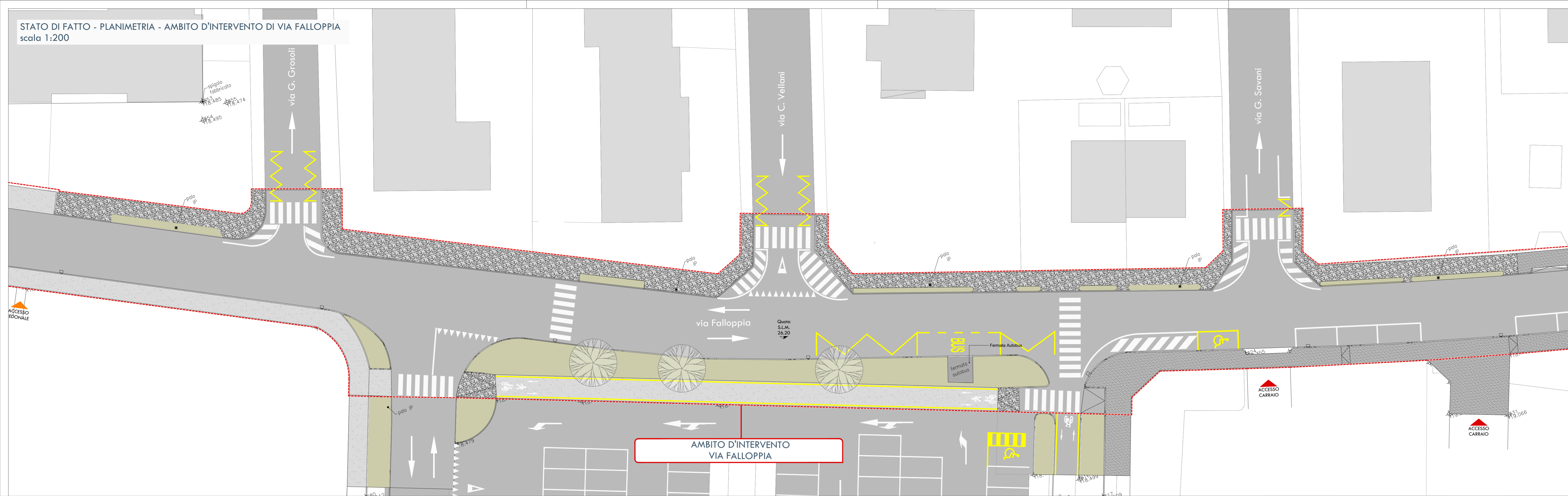
STATO DI FATTO - PLANIMETRIA - AMBITO D'INTERVENTO DI VIA FALLOPPA scala 1:200
