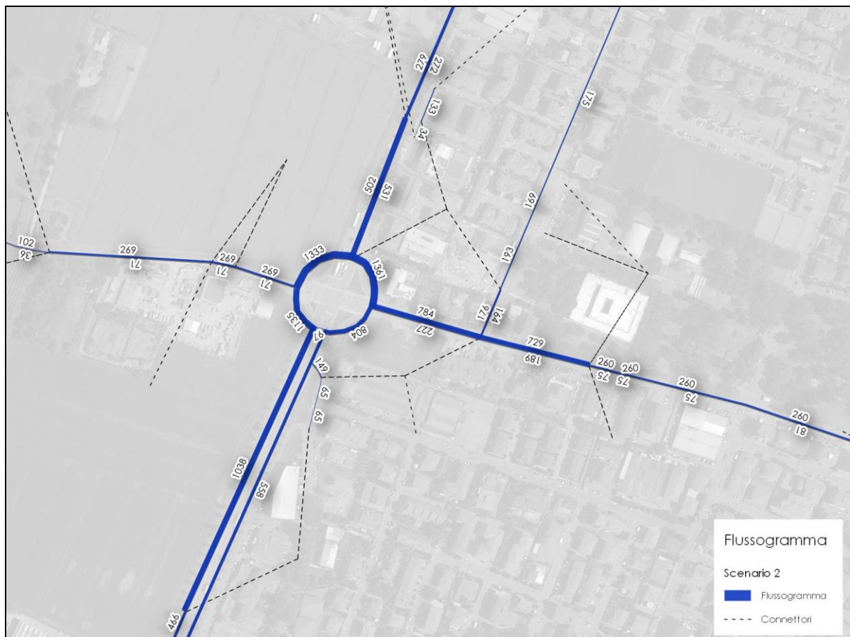
Figura 13 - Flussogramma dei volumi assegnati nello scenario di progetto 2
