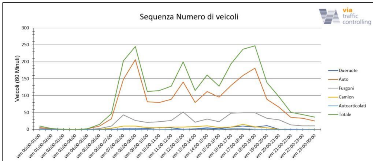
Figura 8 Andamento orario del traffico di venerdì 17 settembre 2021 sulla sezione di Via Quattro Pilastri
