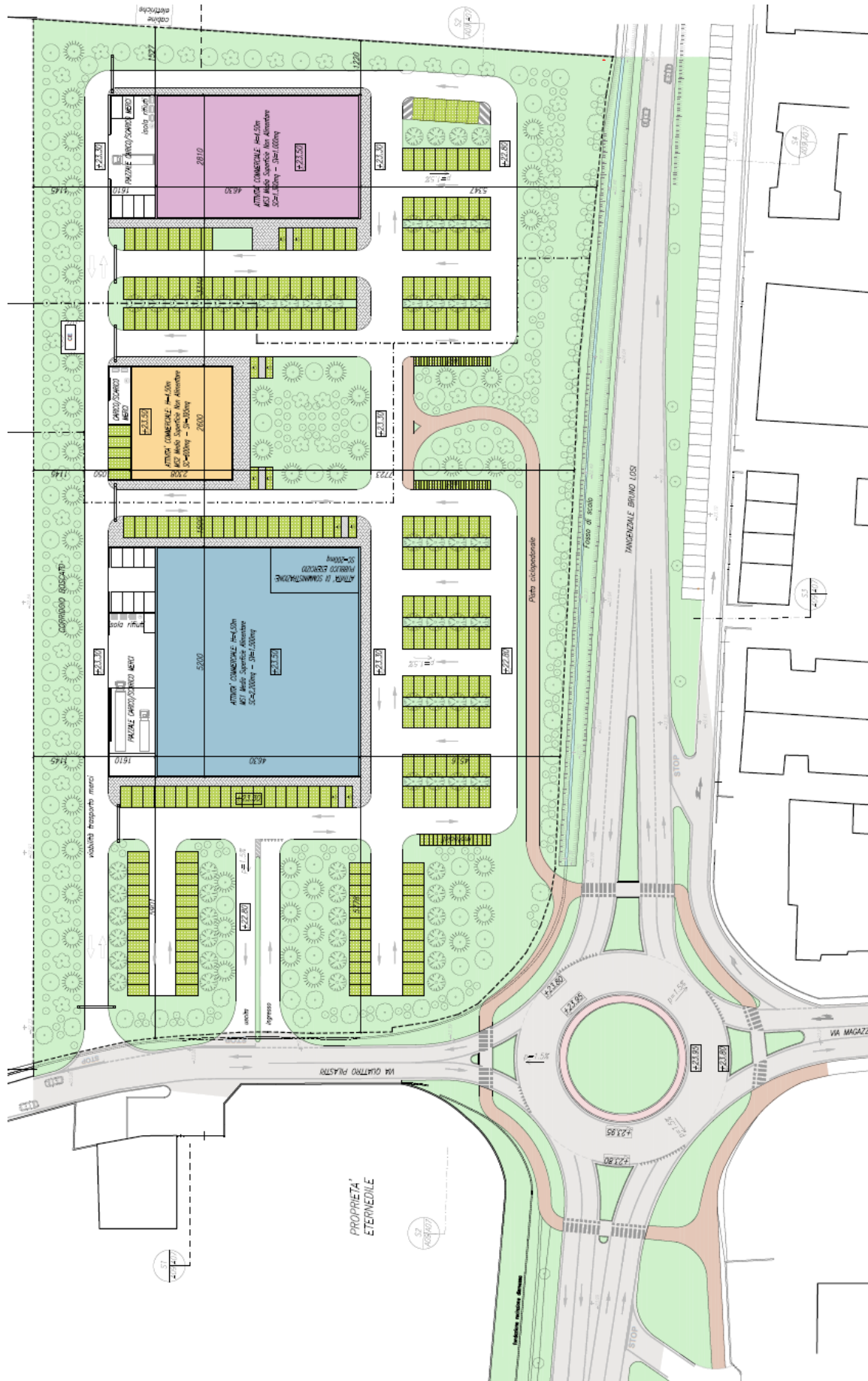
Figura 3 - Planivolumetrico di progetto
