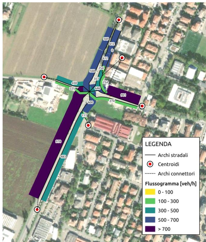
Figura 4 - Flussogramma risultante dal modello di microsimulazione
