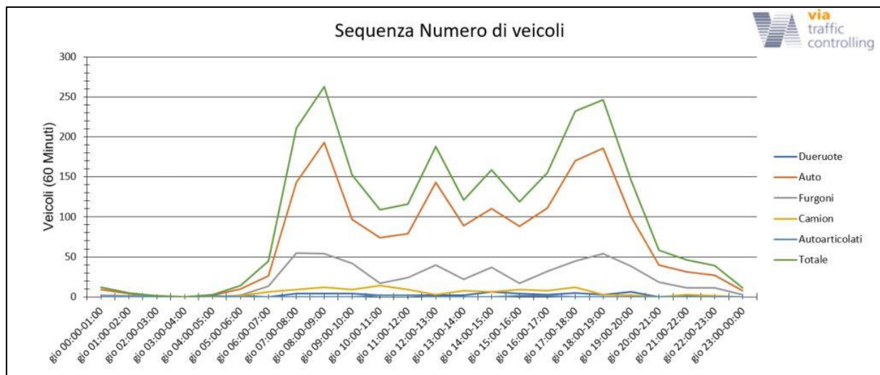
Figura 7 Andamento orario del traffico di giovedì 16 settembre 2021 sulla sezione di Via Quattro Pilastri
