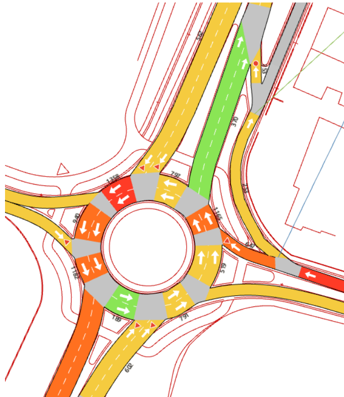
Figura 7 - Flussogramma saturazione della rotatoria (immagine estratta dal software di microsimulazione)
