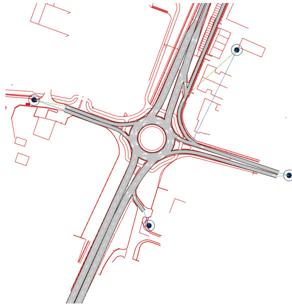
Figura 2 -- Immagine del modello di microsimulazione implementato per la verifica di funzionalità della rotatoria
