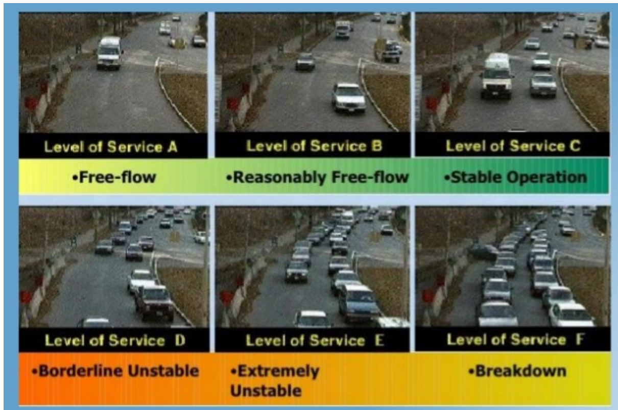
Figura 3: Condizioni di deflusso e relativi livelli di servizio
