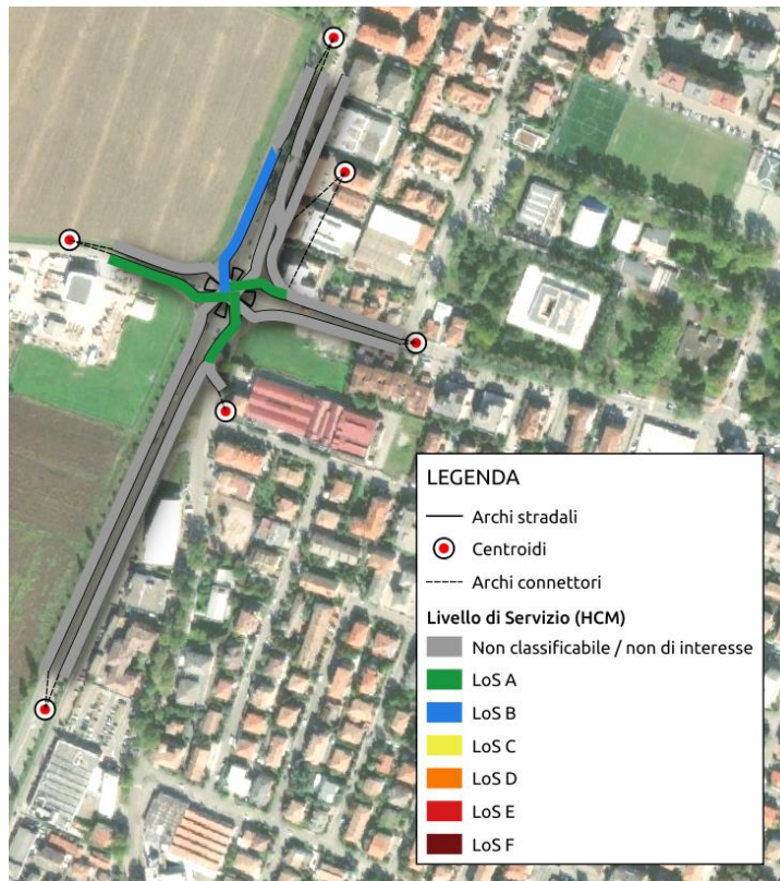
Figura 5 – Livello di servizio sui rami di accesso alla rotatoria risultante dal modello di microsimulazione
