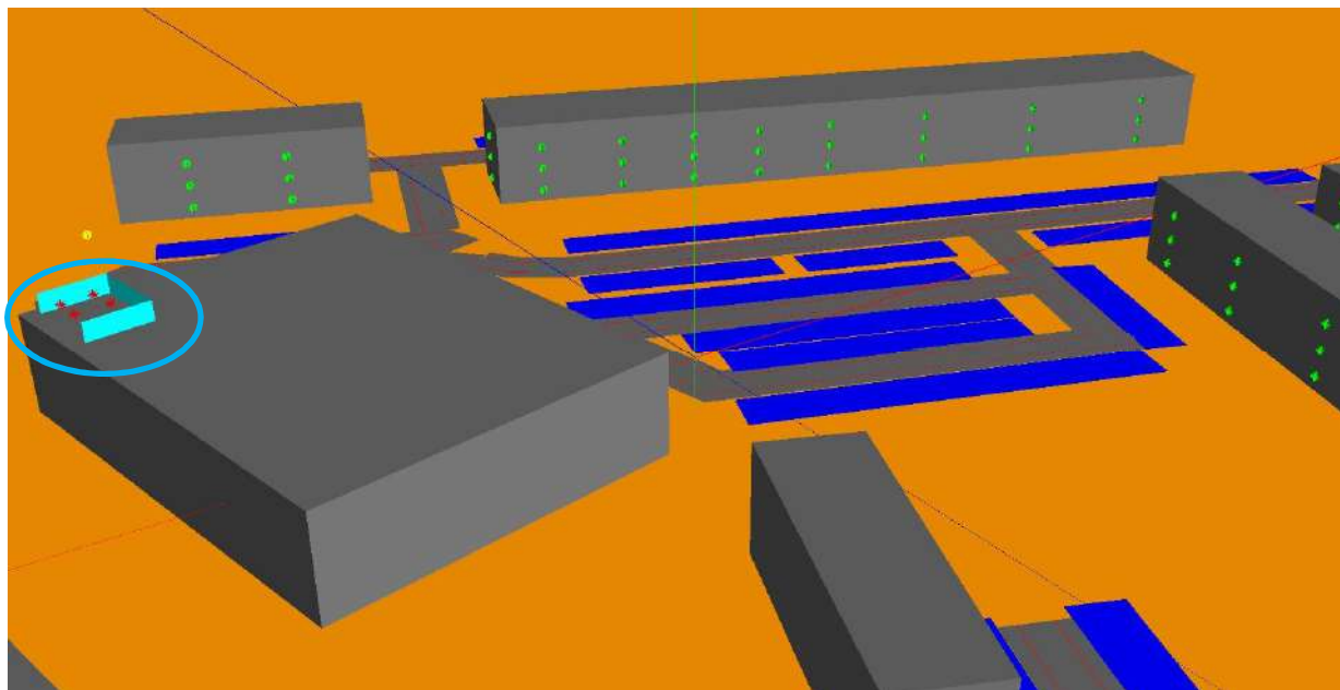
Figura 14 barriera di mitigazione acustica delle sorgenti impiantistiche in copertura esercizio commerciale
