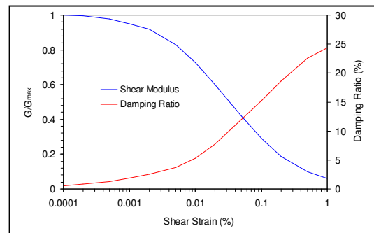
Fig. 13 - Variazione di G e D Sabbie. (Seed & Idris - Media)
