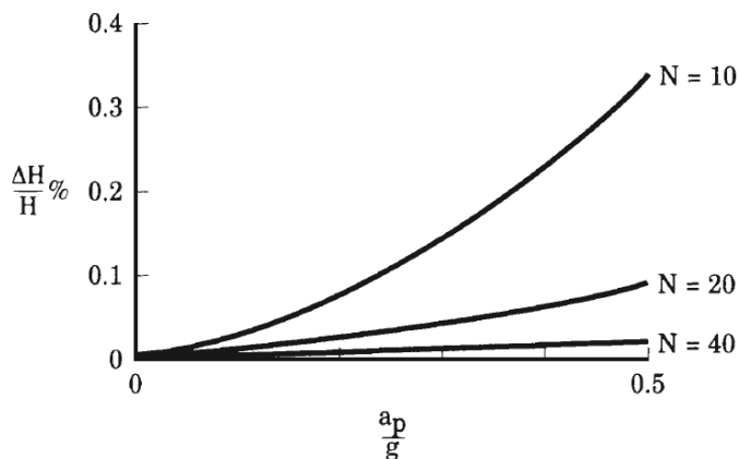
Fig. 21 - Figura per il calcolo dei cedimenti in terreni granulari non saturi (Krinitzsky et al. 1993)
